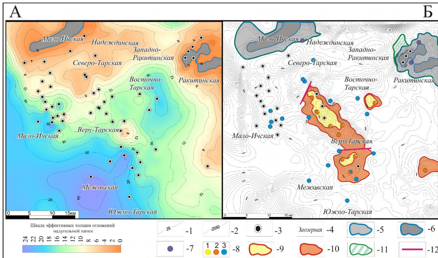
Рис. 5. Карта эффективных толщин отложений (А), карта распределения залежей УВ и нефтегазоперспективных объектов (Б) надугольной пачки горизонта Ю 1 васоганской свиты
