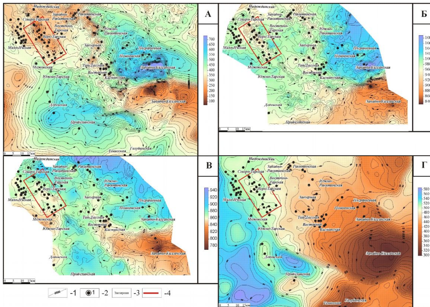
Рис. 2. Карты изобахит отложений Межовского мегамыса
