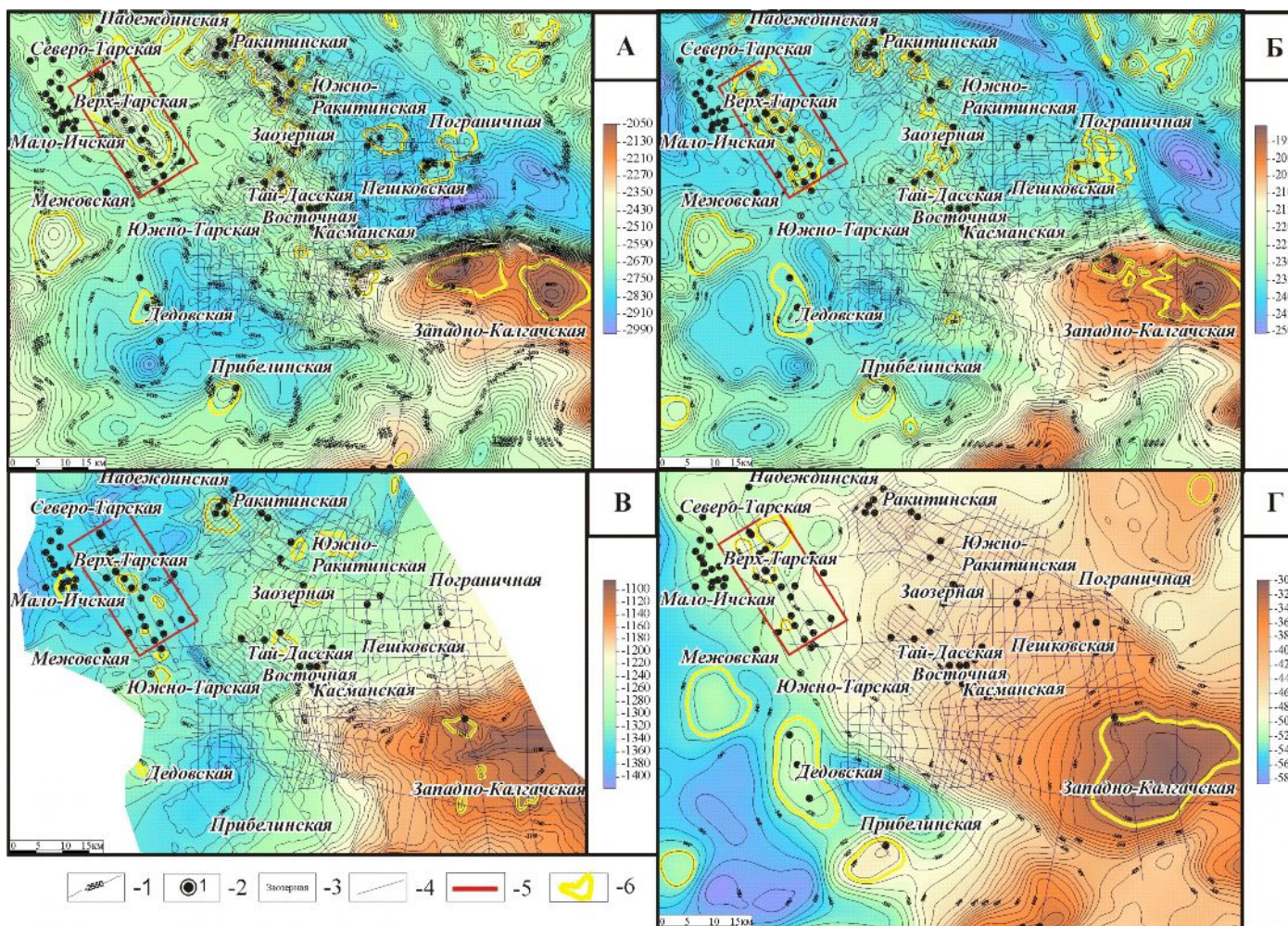
Рис. 1. Структурные карты Межовского мегабасина
