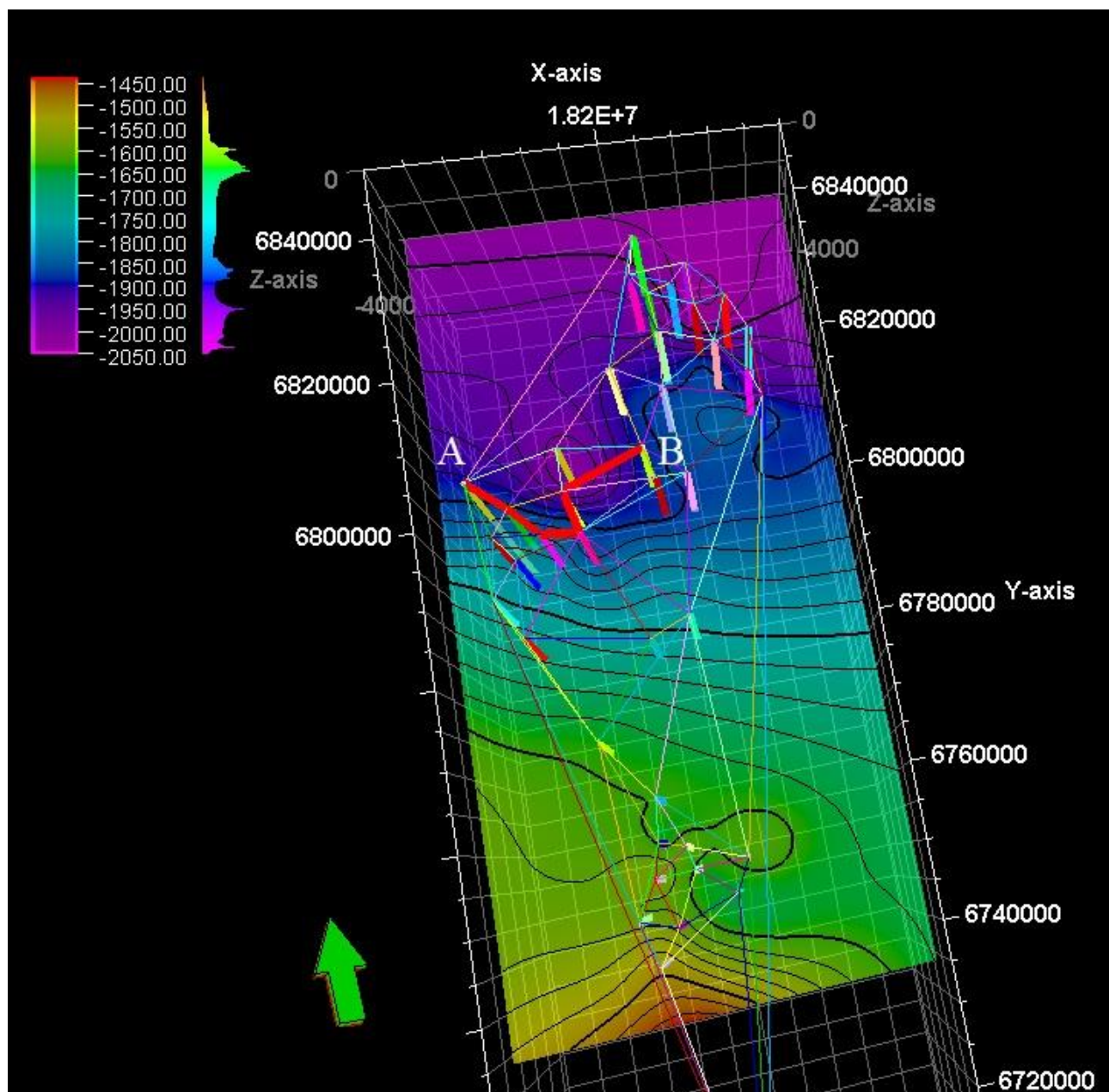
Рис. 1. Границы участка и расположение скважин «Чаяндинского» проекта на подложке структурной карты кровли пласта В 10
