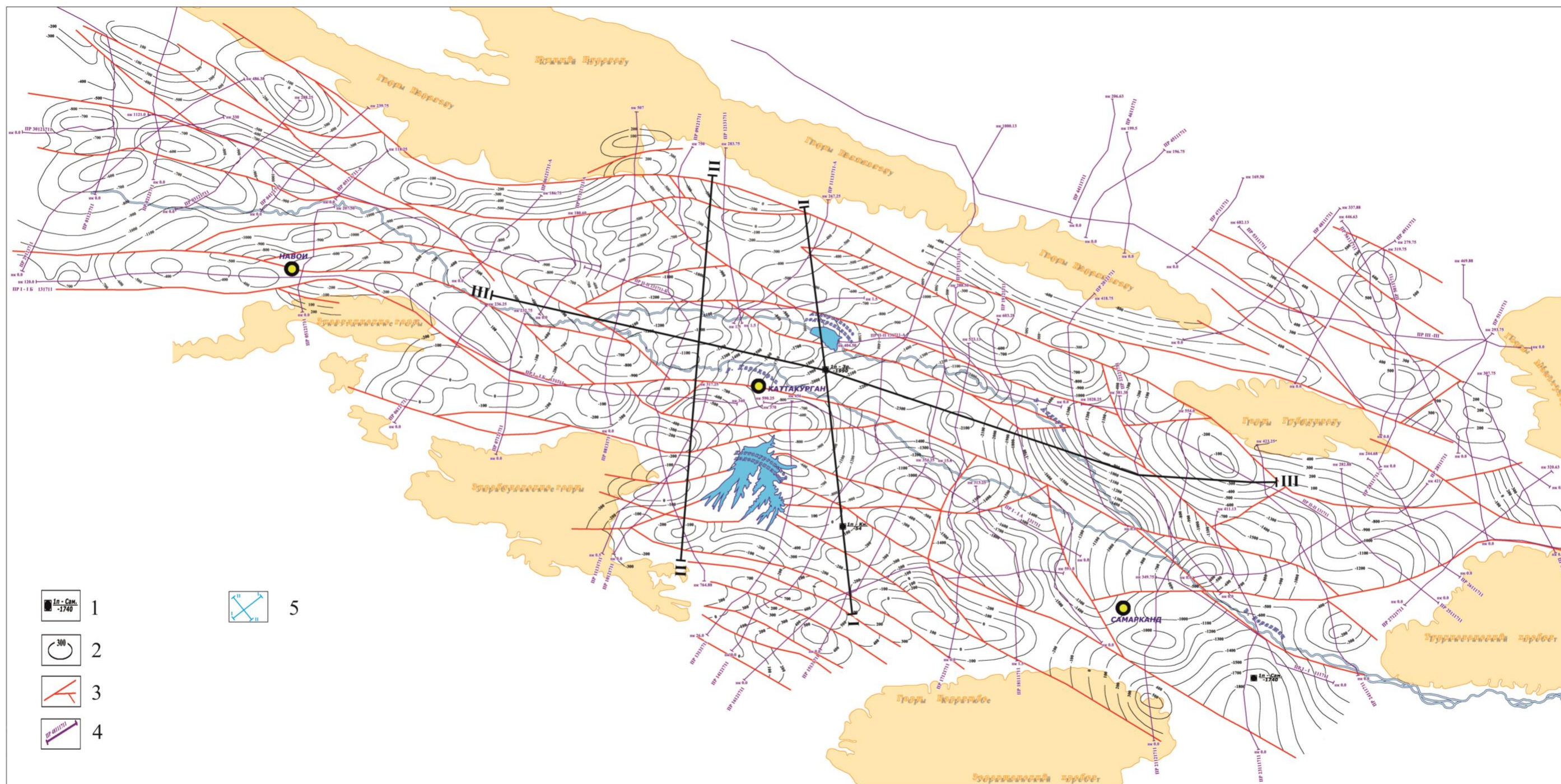
Рис. 1. Схематическая структурная карта по кровле отражающего горизонта T 8 (Pz) Зарафшанской впадины (составила Л.Н. Сафанова, 2017 г.)
