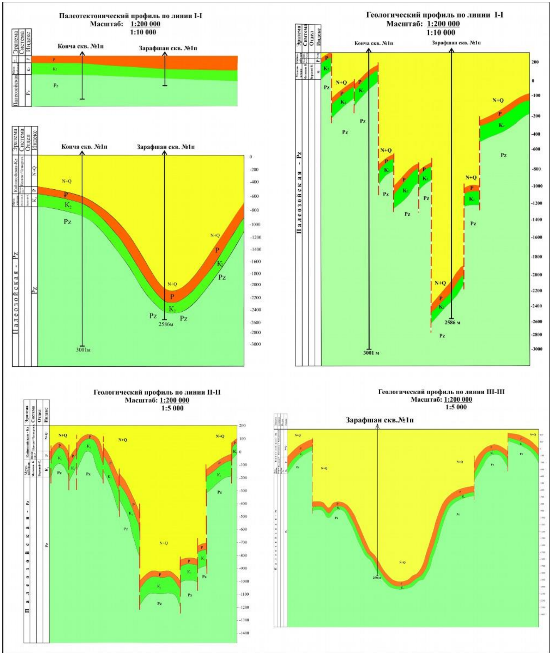
Рис. 2. Палеотектонический и геологические профили по линии (I-I, II-II, III-III) Зарафшанской впадины (составил Б.И. Хожиев, 2018 г.)
