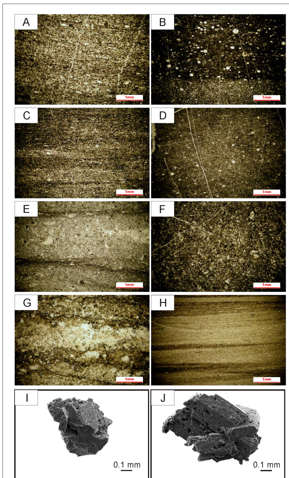
Рис. 3. Фото шлифов и минеральных агрегатов из нижней части воркашорской свиты
