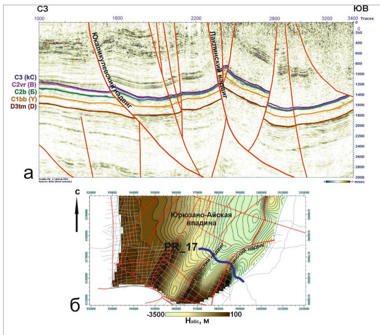
Рис. 12. Юкаликулевский и Лаклинский надвиги на фрагменте сейсмического профиля PR-17 (а) и структурная карта по отражающему горизонту C2vr (б)
