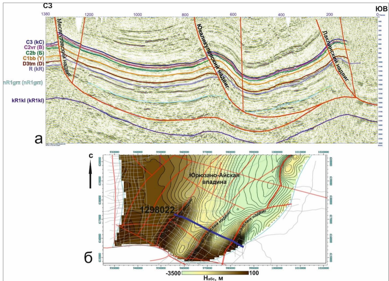
Рис. 11. Месягутовский, Юкаликулевский и Лаклинский (Апутовский) надвиги на сейсмическом профиле 1298022 (а) и структурная карта по отражающему горизонту C2vr (б)
