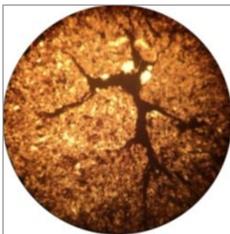
Рис. 24. Фото глины алевритистой с небольшим количеством обломков песчаной размерности, раскристаллизованной в гидрослюду с углефицированным растительным детритом Порода непористая, нетрециноватая. Ник.-, ув. 9x15.
