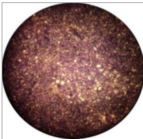
Рис. 3. Фото аргиллита углистого с линзами алевролита, с углефицированным растительным детритом
