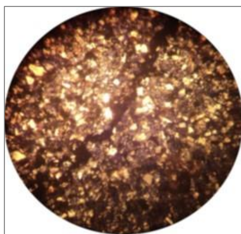
Рис. 4. Фото алевролита песчанистого, сильно глинистого, полевошпат-кварцевого с цементом глинистым, кремнисто-глинистым, с углефицированным растительным детритом
