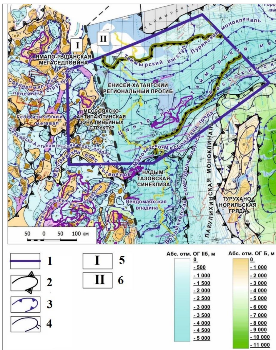
Рис. 2. Фрагменты тектонической схемы зоны сочленения Енисей-Хатангского регионального прогиба с Мессояхско-Антипаутинской зоной линейных структур
