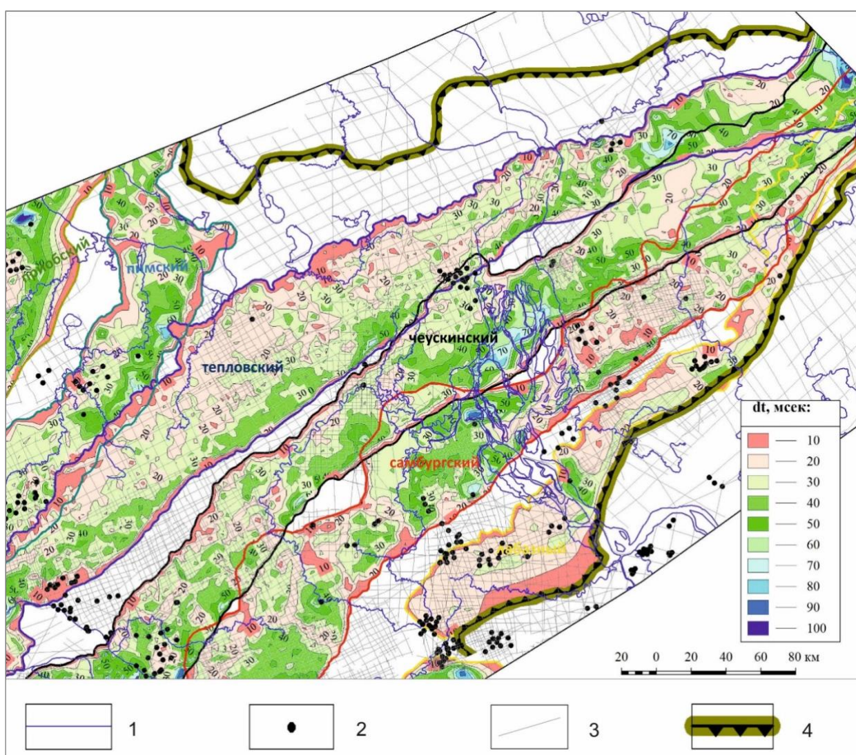
Рис. 5. Схема временных толщин глубоководных отложений по крупным сеймостратиграфическим комплексам
