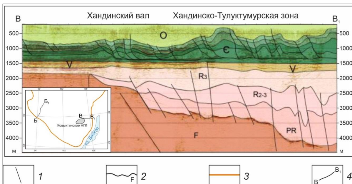
Рис. 5. Глубинный разрез через юго-восточную часть Сибирской платформы [Мисюркеева, 2022]
